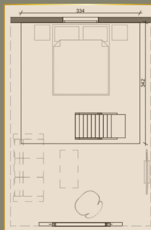
OSNOVA POTKROVLJA
