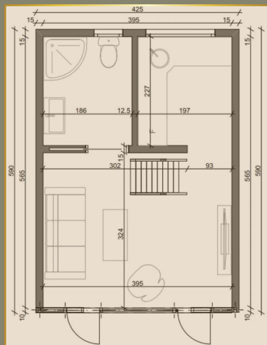
OSNOVA PRIZEMLJA
