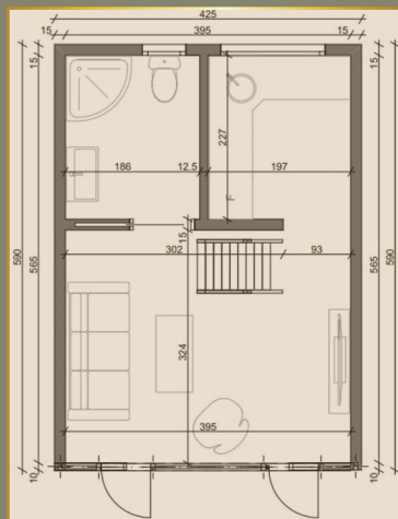
OSNOVA PRIZEMLJA
